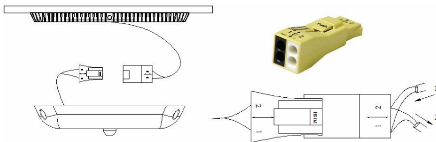
Рисунок 4 – Подключение светильника.
